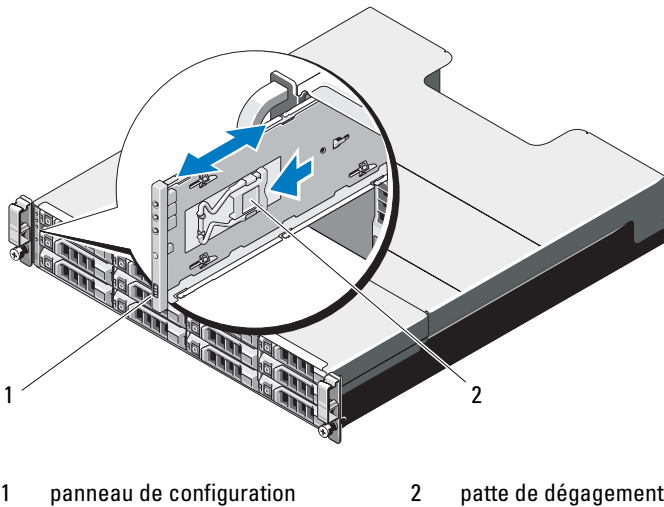
Figure 16-13. Retrait et installation du panneau de commande du PowerVault MD3600i
