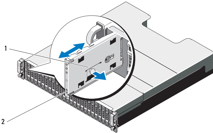
Figure 16-14. Retrait et installation du panneau de commande du PowerVault MD3620i
