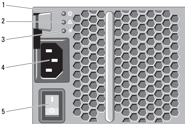
Figure 2-6. Codes et fonctionnalités des voyants d'alimentation
