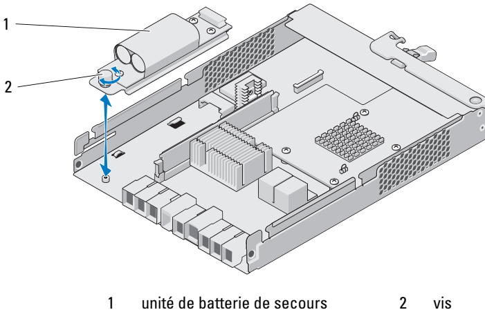
Figure 16-10. Retrait et installation de l'unité de batterie de secours du module de contrôleur RAID
