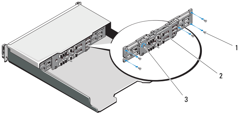
Figure 16-16. Retrait et installation du fond de panier du PowerVault MD3600i
