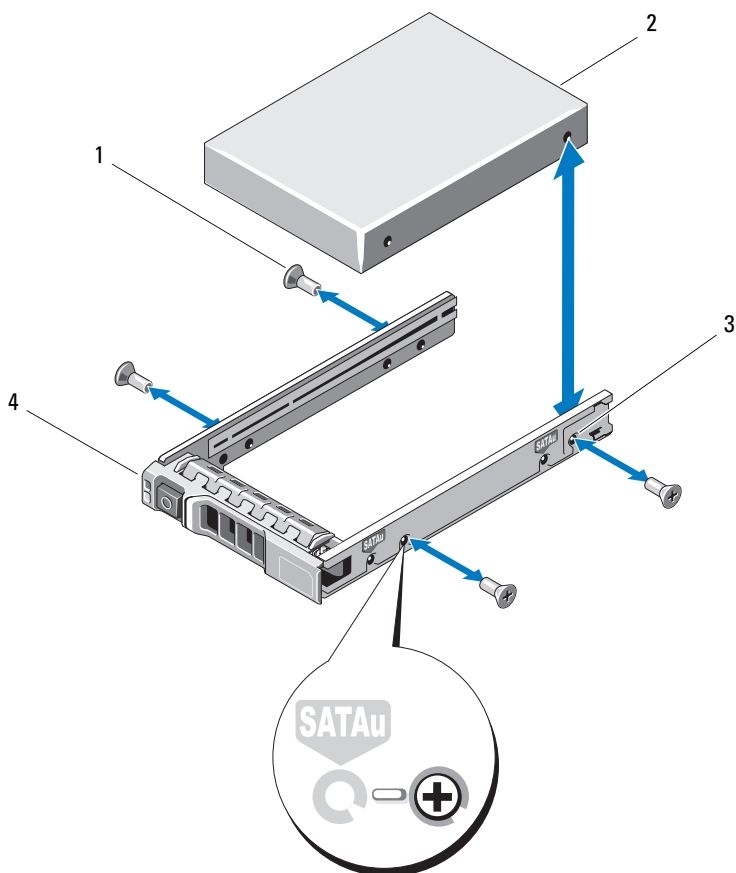
Figure 16-6. Retrait et installation d'un disque dur dans un support de disque de 2,5 pouces
