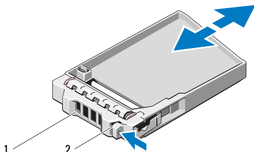
Figure 16-3. Retrait et installation d'un cache de lecteur de disque dur 3,5 pouces (MD3620i uniquement)
