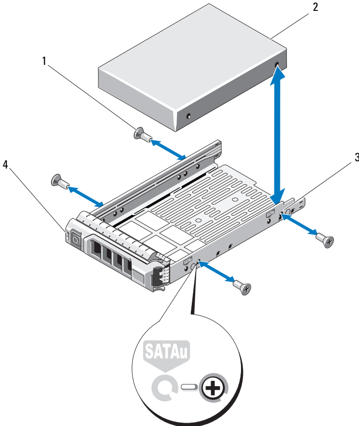
Figure 16-5. Retrait et installation d'un disque dur dans un support de disque de 3,5 pouces
