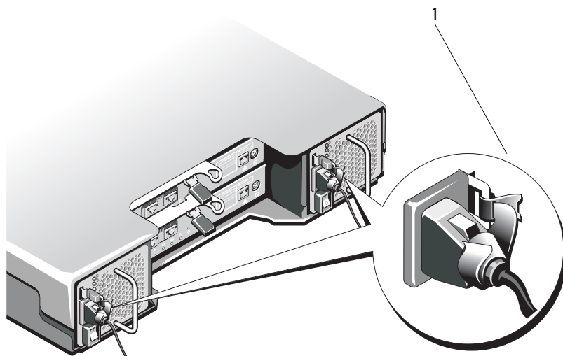
Figure 16-12. Fixation du câble d'alimentation
