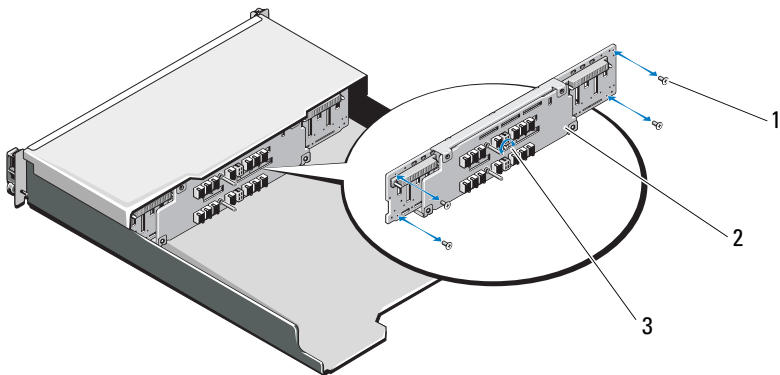
Figure 16-17. Retrait et installation du fond de panier du PowerVault MD3620i
