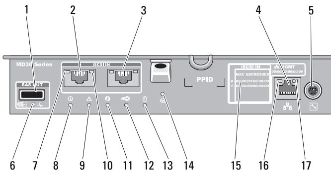
Figure 3-1. Module de contrôleur RAID iSCSI série MD3600i
