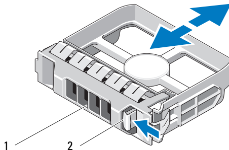
Figure 16-2. Retrait et installation d'un cache de lecteur de disque dur de 3,5 pouces
