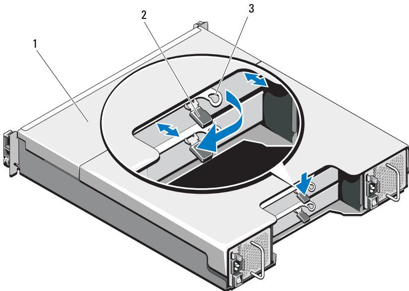
Figure 16-8. Retrait et installation d'un module de contrôleur RAID
