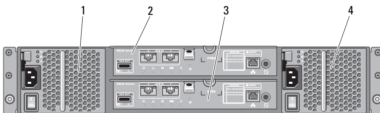
Figure 2-4. Voyants et caractéristiques du panneau arrière : Matrice de stockage de série Dell PowerVault MD3600i
