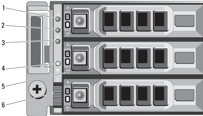
Figure 2-1. Voyants et fonctions du panneau avant — Dell PowerVault MD3600i
