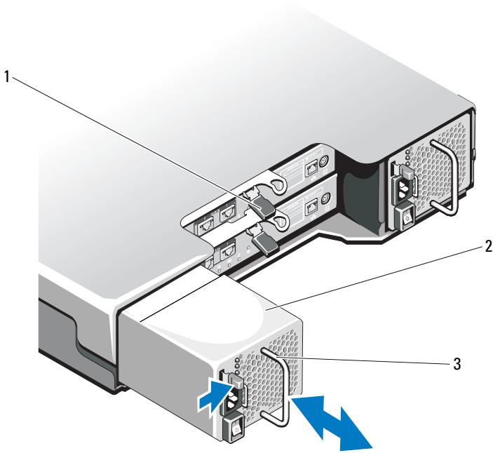
Figure 16-11. Retrait et installation d'un module de bloc d'alimentation/ventilateur de refroidissement
